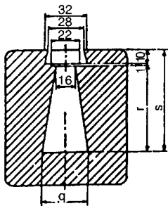
Prerez EE
