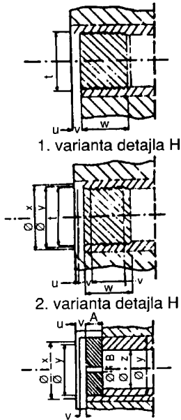
Detajl H
